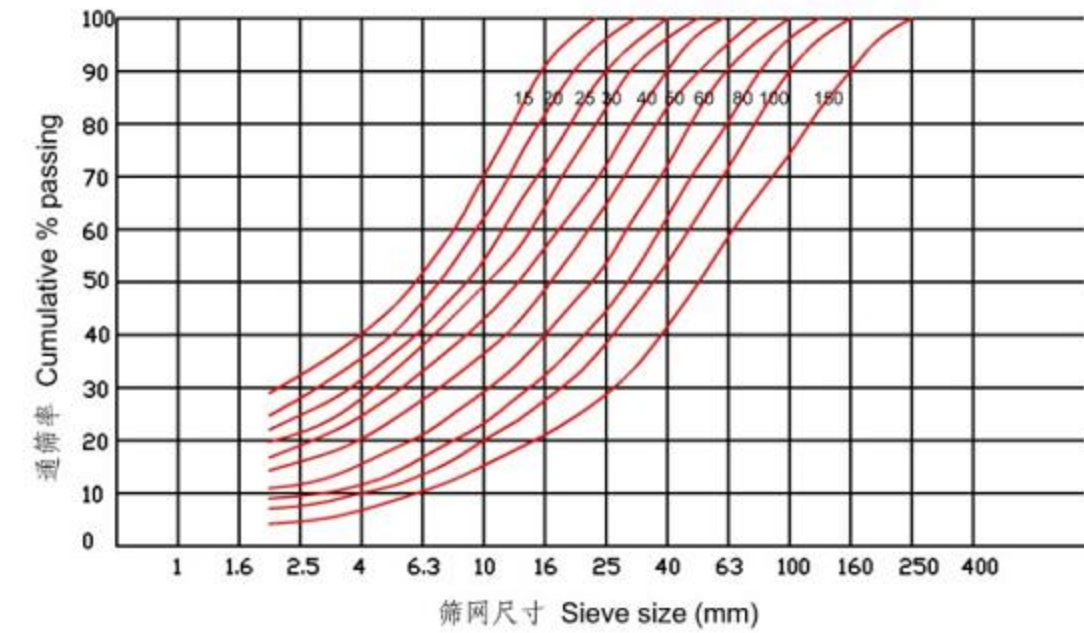
产品粒度曲线 Production curves
